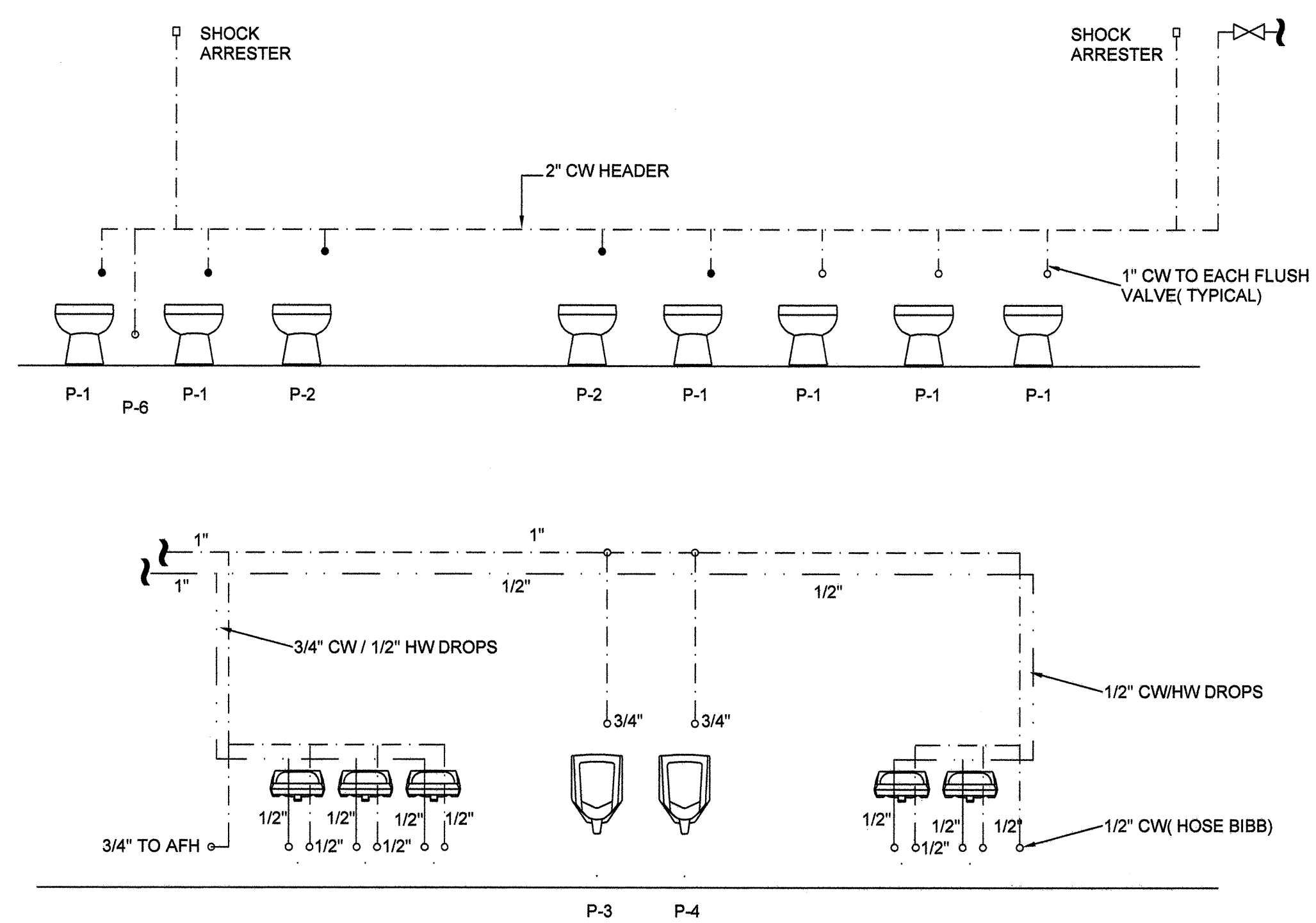
5 WATER RISER - TOILET 137 & 138 P-2 N.T.S.
