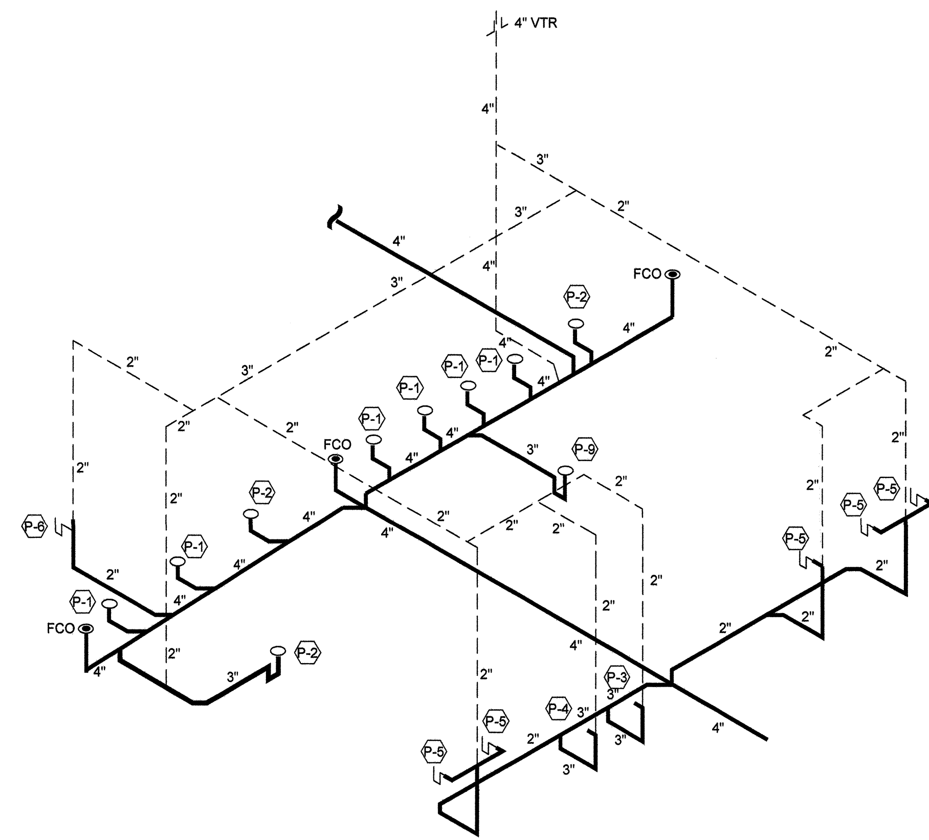
6 DWV RISER DIAGRAM - TOILET 137 & 138 P-2 N.T.S.
