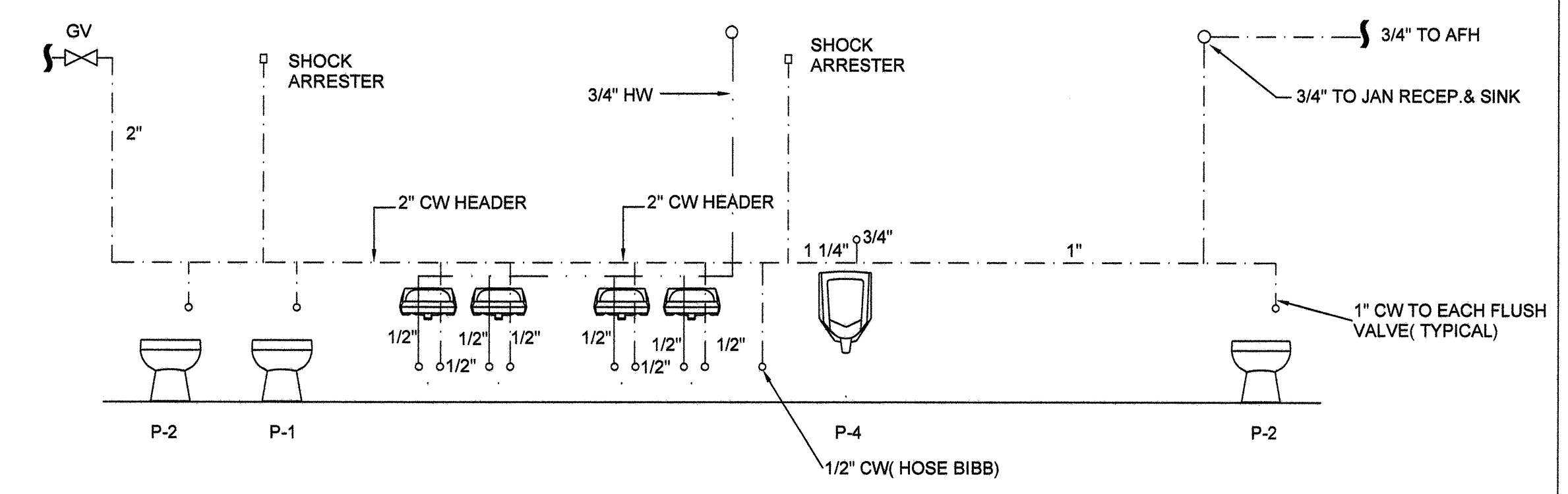
4 WATER RISER - TOILET 118 & 119 P-2 N.T.S.
