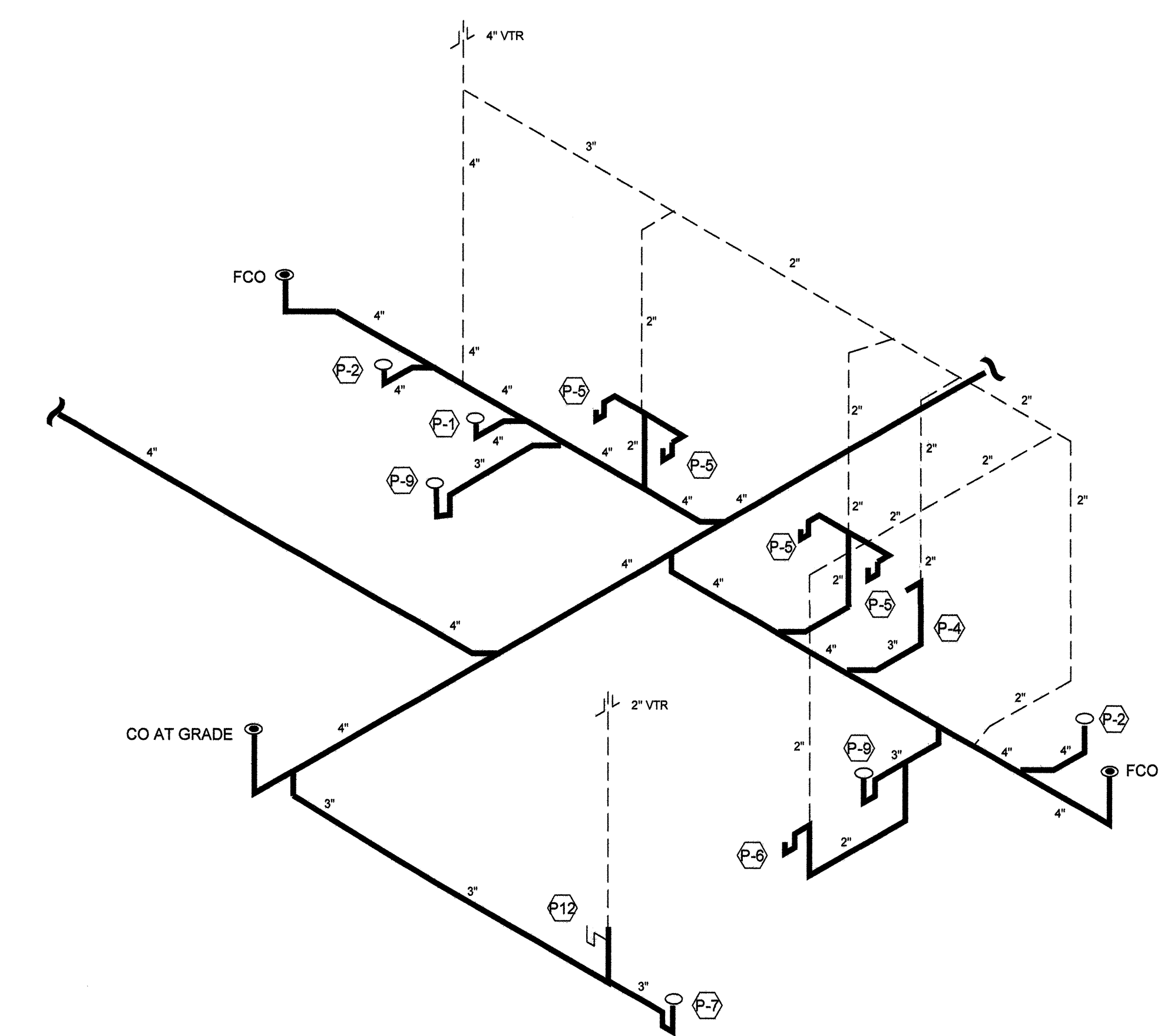
7 DWV RISER DIAGRAM - TOILET 118 & 119 P-2 N.T.S.
